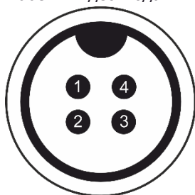
Схема контактов разъёма 4 PIN (папа) кабеля видеовхода AV IN3
